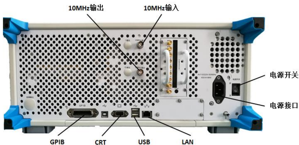
图 3.2 后面板说明
