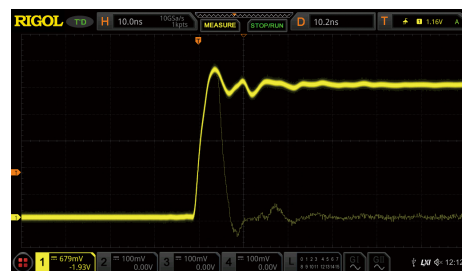
高刷新率模式下捕获偶发异常信号
