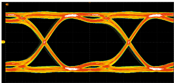
使用600 MHz带宽和1 GHz带宽分别对1 Gb/s信号进行眼图观测
