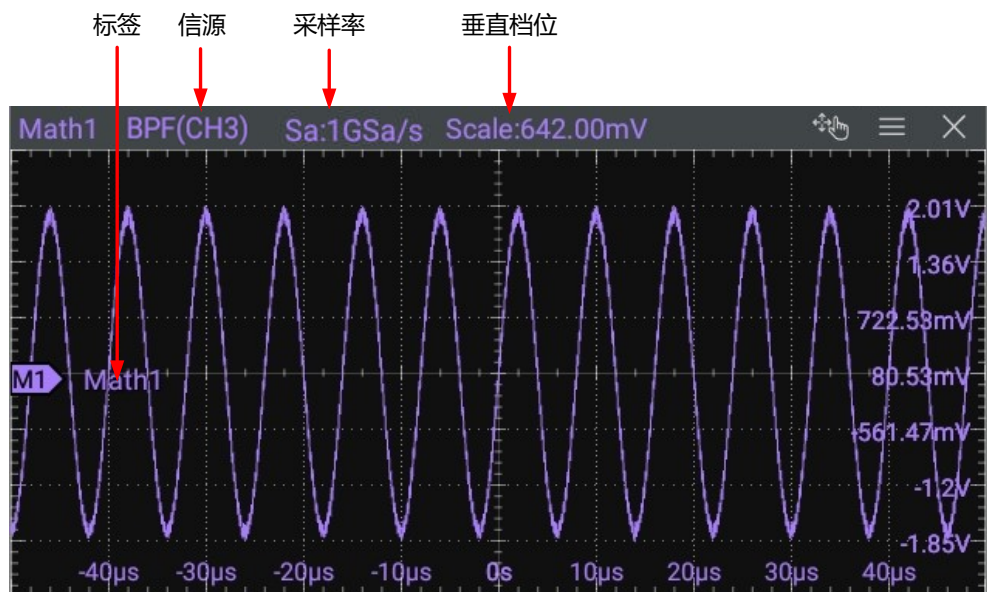
图 9.13 运算结果显示窗口
