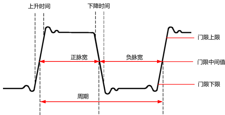
图 10.1 时间参数
