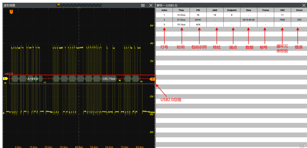
图 17.27 USB2.0 解码事件表
