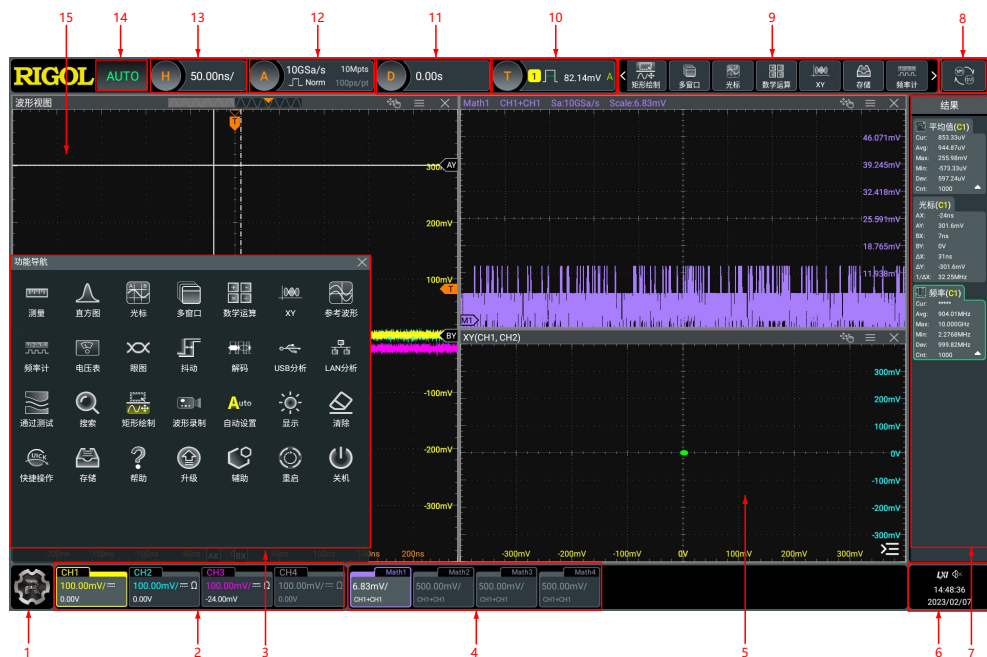
图 4.12 DS80000 用户界面
