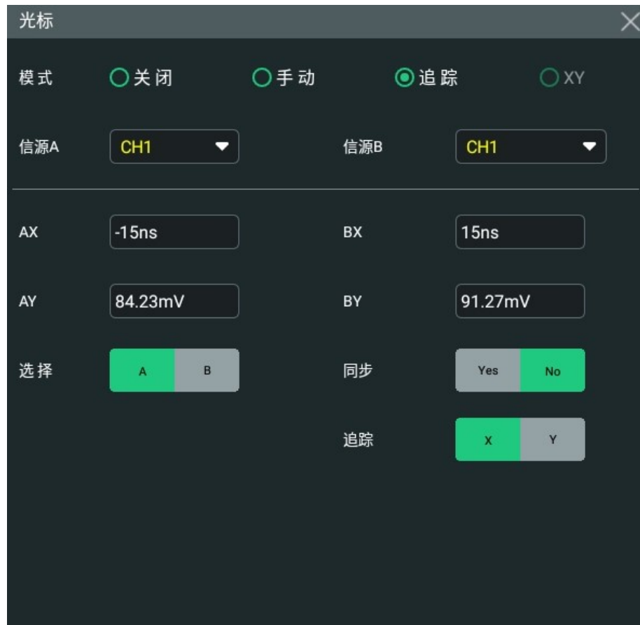
图 10.12 追踪模式光标设置菜单
