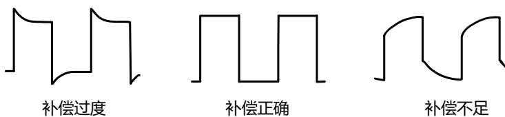
图 4.9 探头补偿
