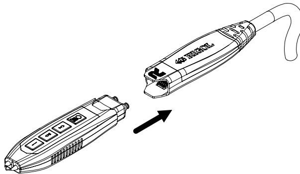
图 4.5 连接探头前端与有源探头放大器
