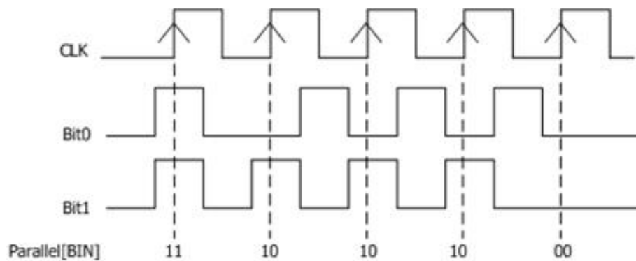
图 17.1 GPIO 解码示意图
