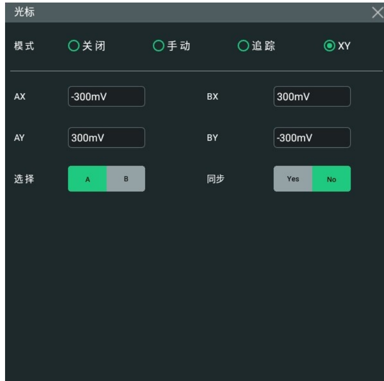
图 10.15 XY 光标
