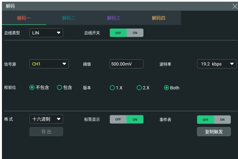
图 17.14 LIN 解码菜单
