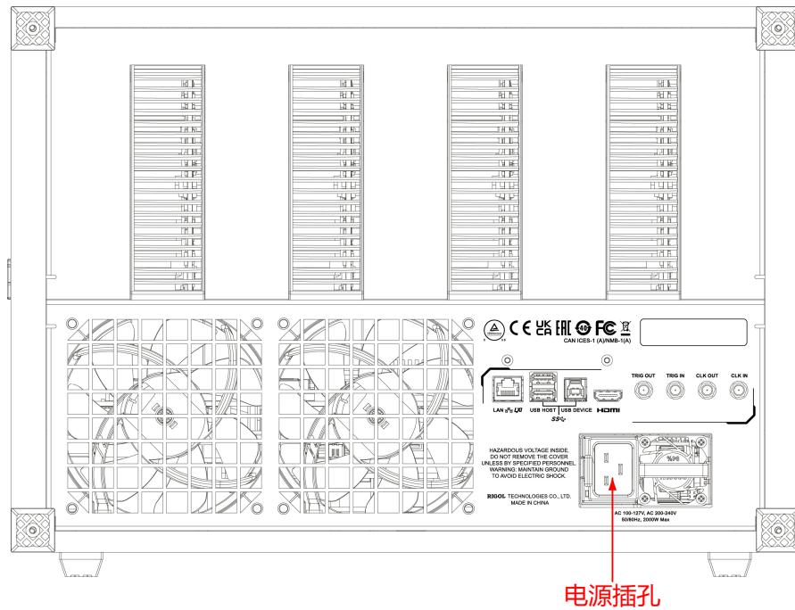
图 4.3 连接电源
