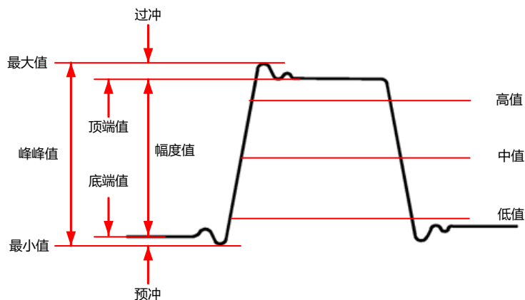
图 10.3 电压参数
