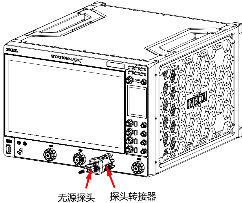
图 4.4 连接无源探头
