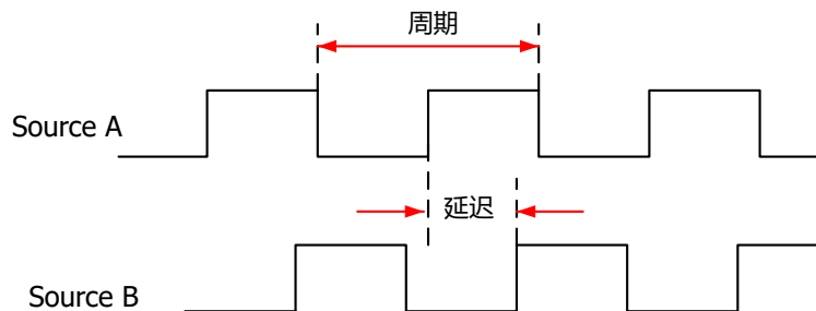
图 10.2 延迟和相位参数
