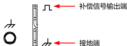
图 4.7 补偿信号
