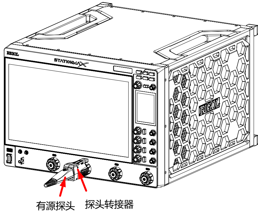
图 4.6 连接有源探头
