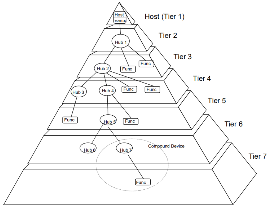
图 17.26 USB 拓扑图
