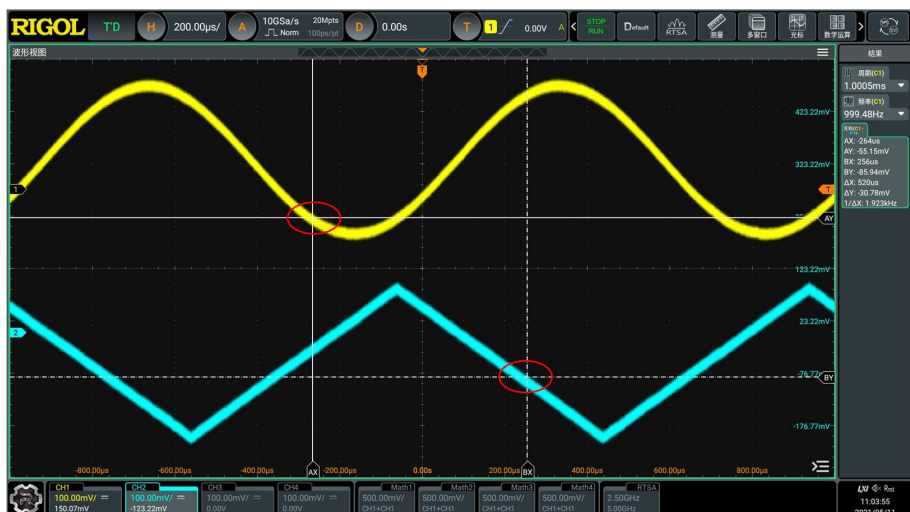
图 10.14 追踪测量 (水平扩展后)
