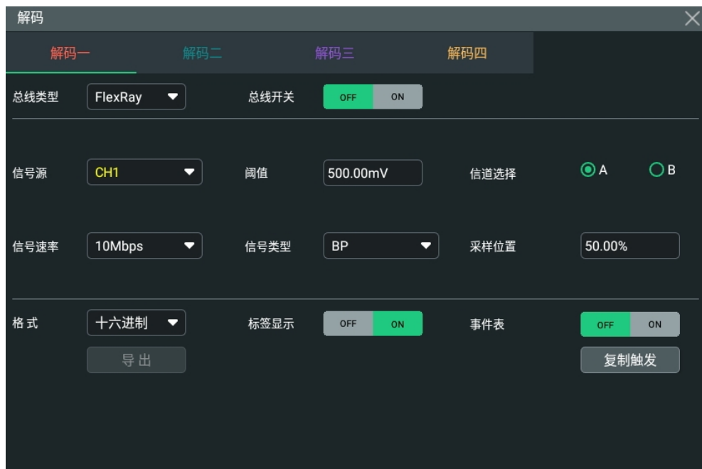
图 17.19 FlexRay 解码菜单
