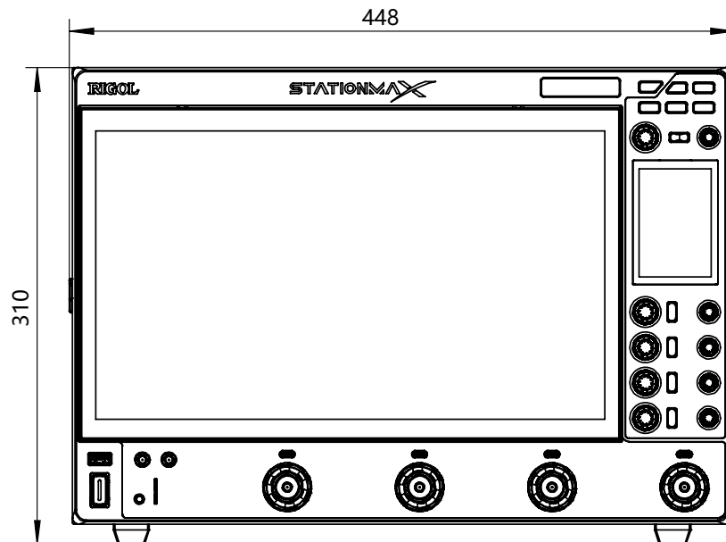
图 4.1 正视图 (单位: mm)
