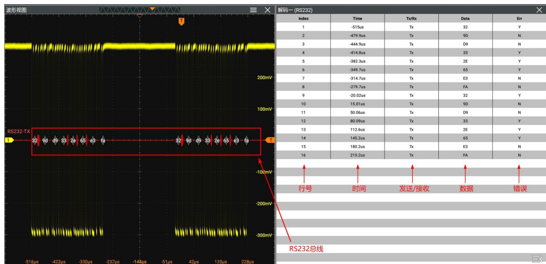
图 17.7 UART/RS232 解码事件表
