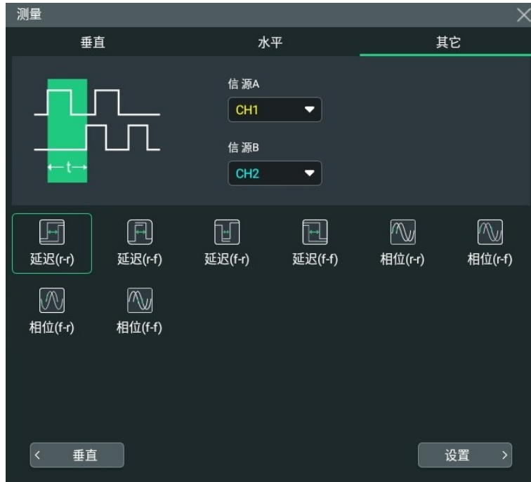
图 10.6 其他测量参数
