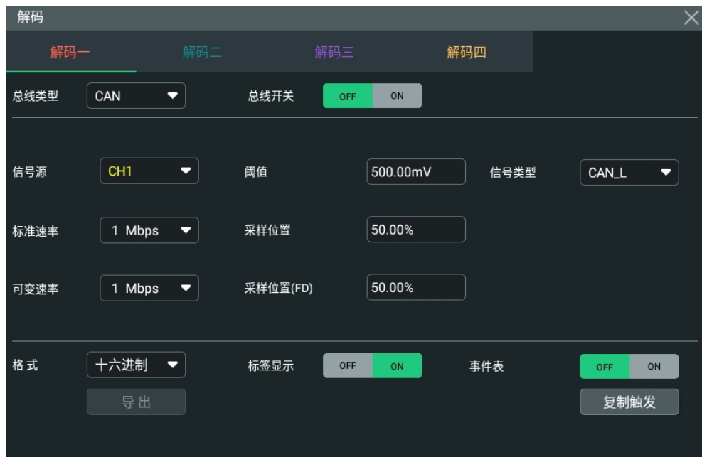
图 17.16 CAN 解码菜单
