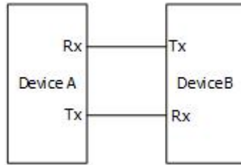
图 17.4 UART/RS232 串行总线示意图
