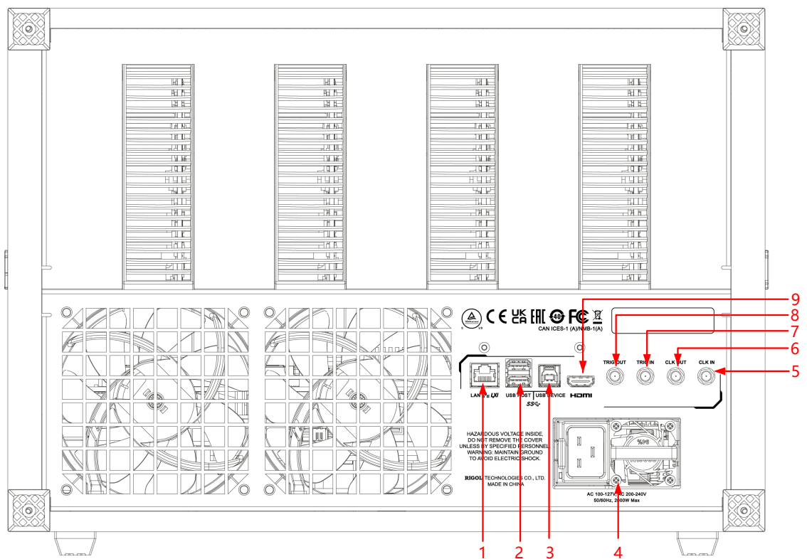
图 4.11 DS80000 后面板
