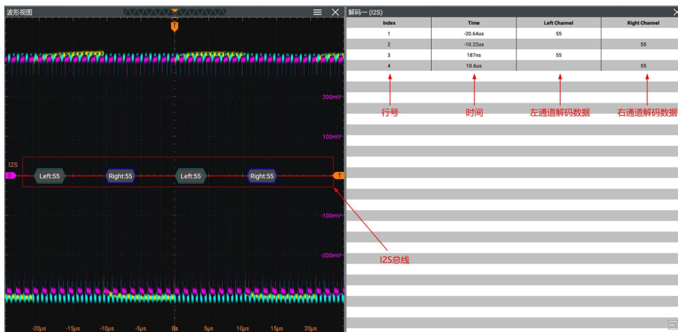
图 17.23 I2S 解码事件表
