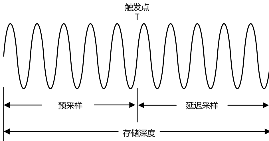
图 7.1 存储深度示意图
