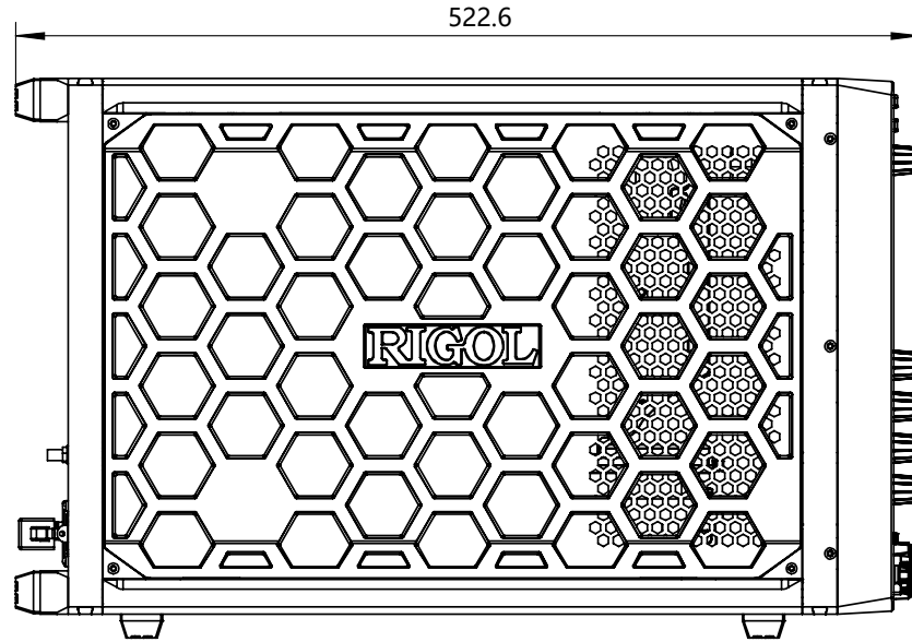
图 4.2 侧视图 (单位: mm)
