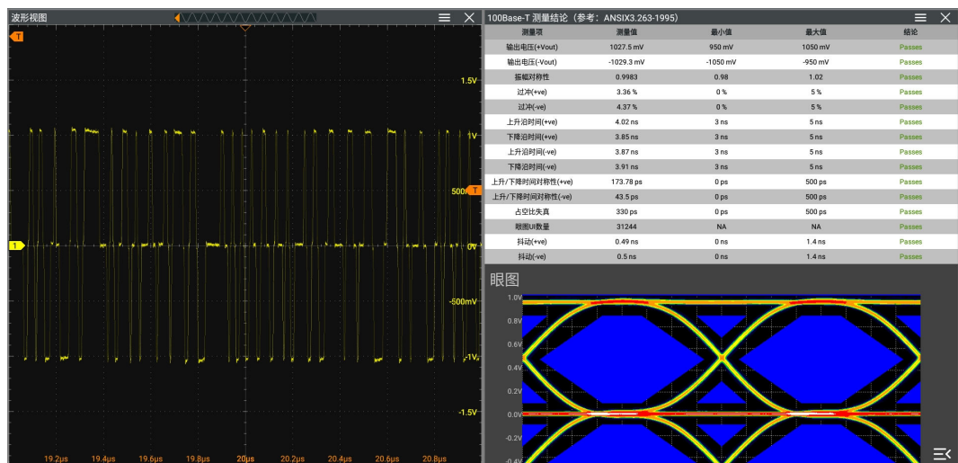
图 18.9 LAN 一致性分析测试报告
