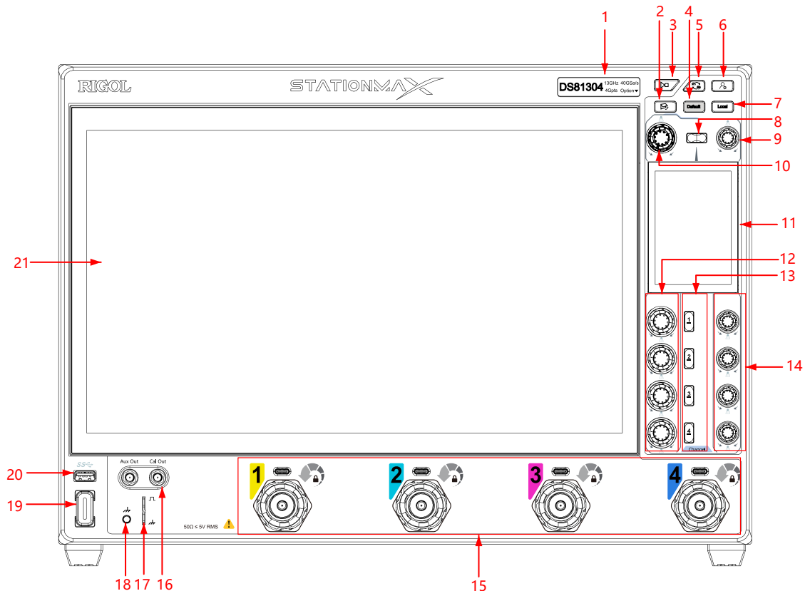
图 4.10 DS80000 前面板
