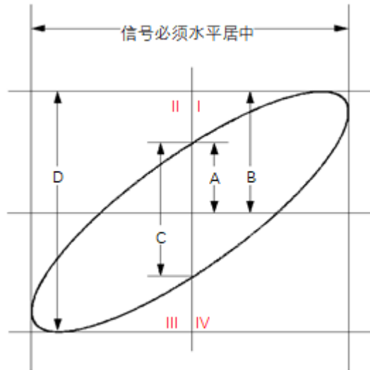
图 7.3 相位差的测量原理图
