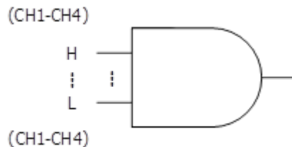
图 8.9 码型触发
