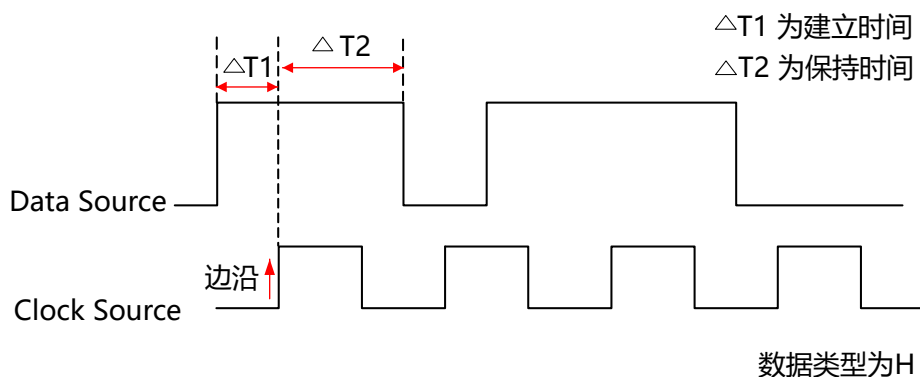
图 8.20 建立保持时间示意图
