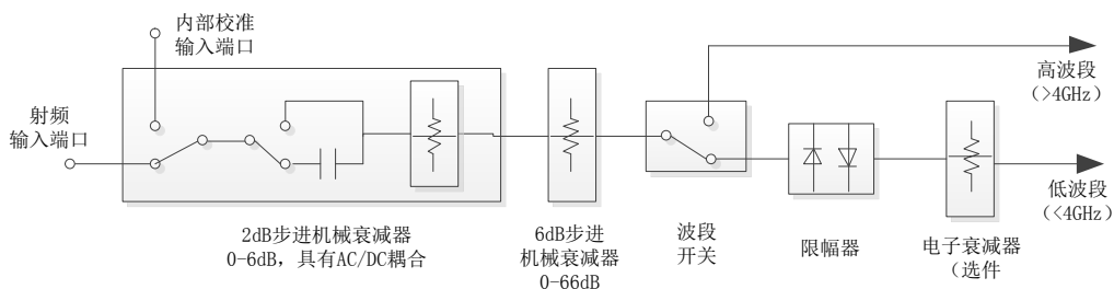
图 4.1 4052 系列信号/频谱分析仪衰减器接连关系
