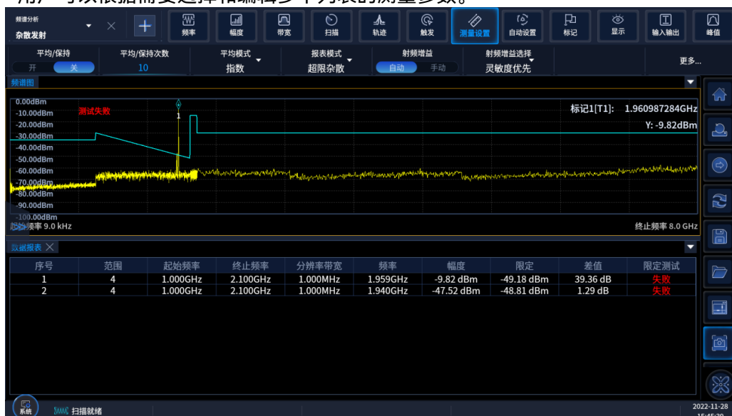
图 4.27 杂散发射测量结果
