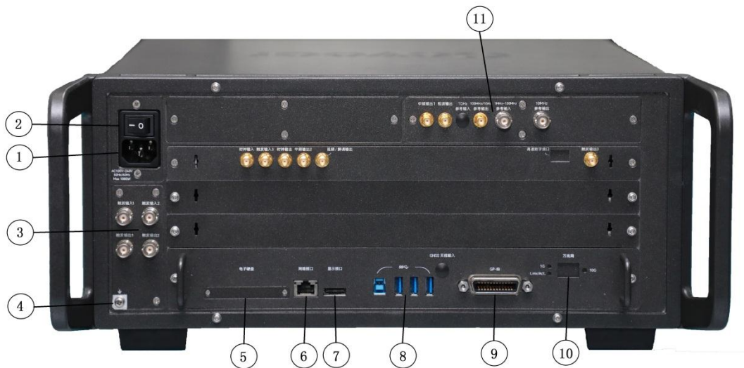
图 3.9 4052 后面板
