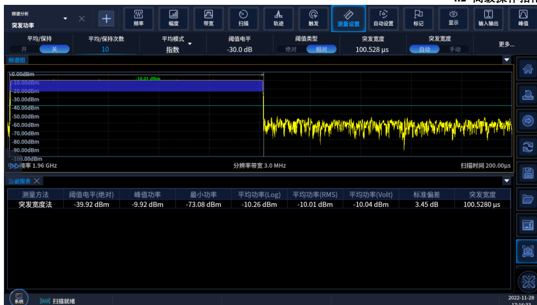
图 4.21 突发功率测量结果
