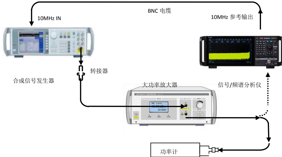
图7.7 最大安全输入电平测试示意图
