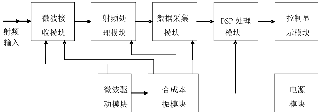
图 6.1 4052 系列信号/频谱分析仪原理框图
