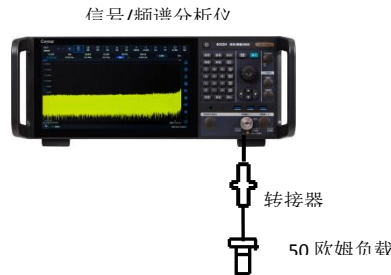
图7.13 显示平均噪声测试示意图
