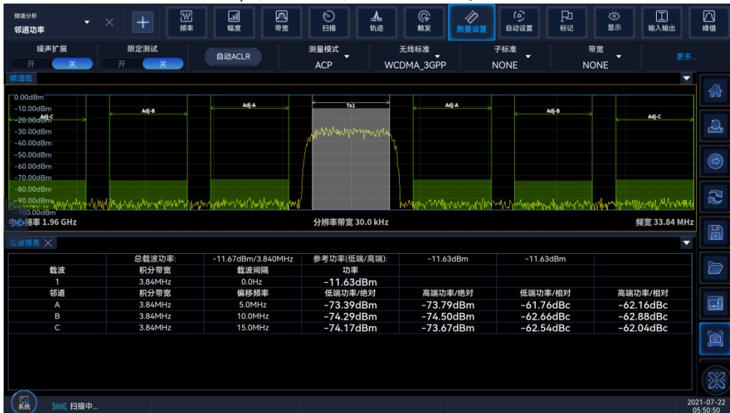
图 4.14 测量第三邻道
