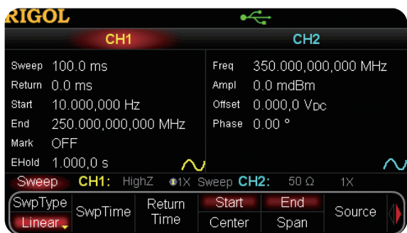
扫频设置
