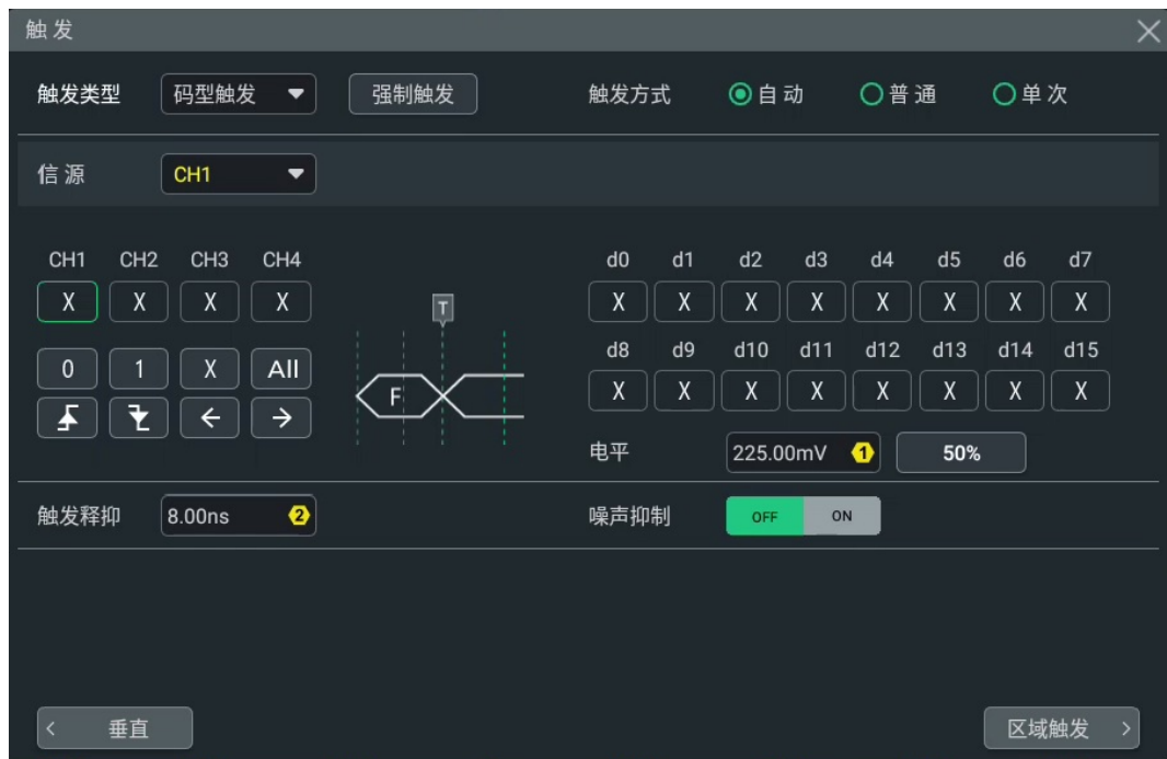
图 8.10 MHO 系列 4 通道型号码型触发配置菜单
