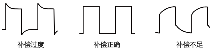
图 4.15 探头补偿
