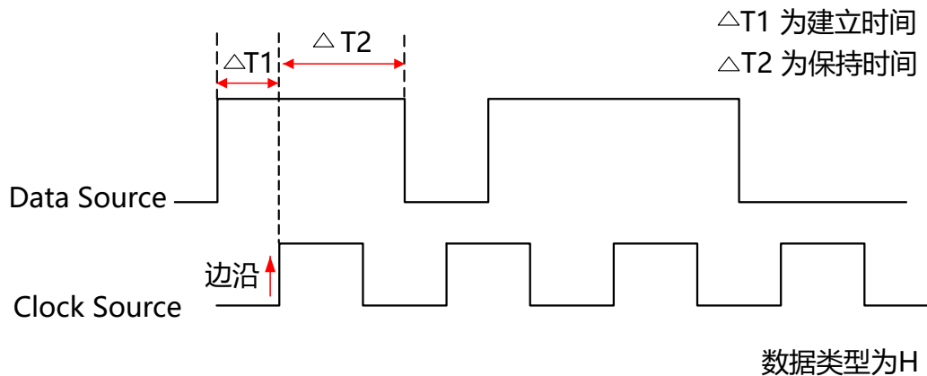
图 8.22 建立保持时间示意图
