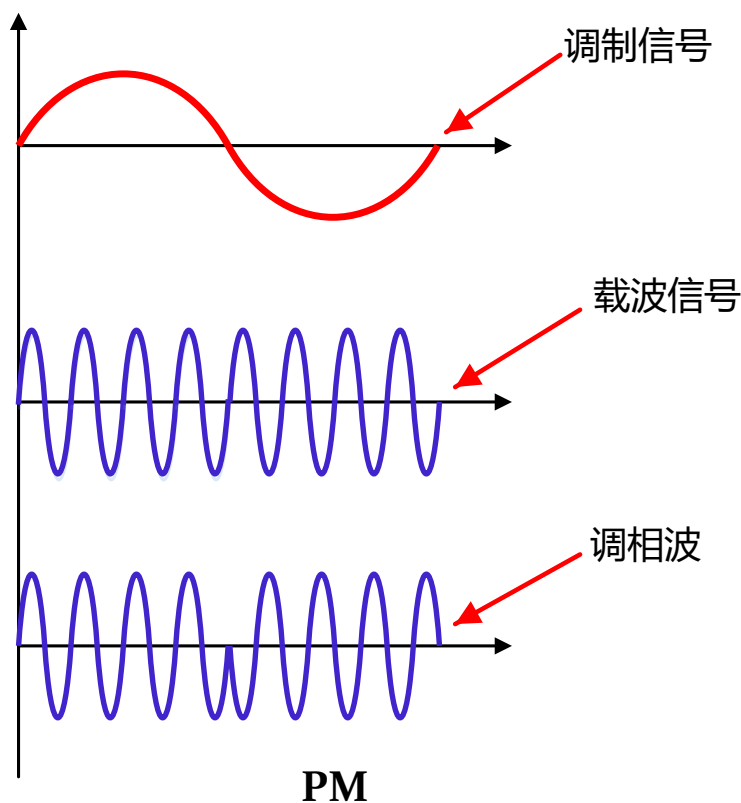
图 14.12 调相
