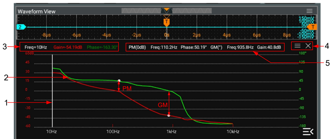
图 15.3 伯德图-波形显示
