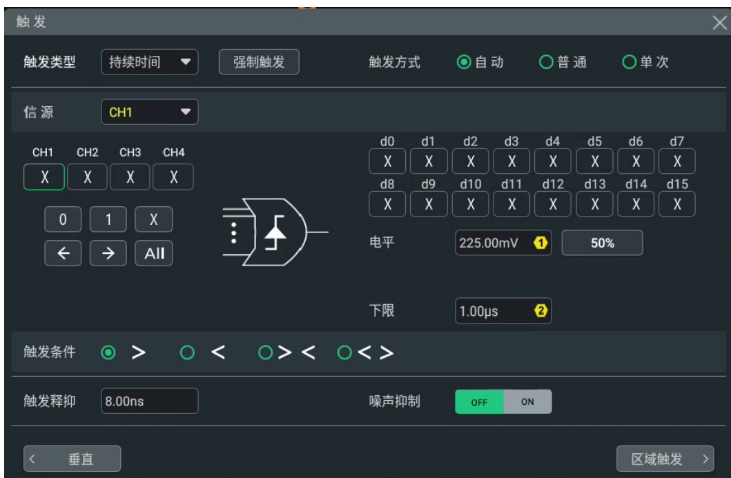
图 8.13 MHO 系列 4 通道型号持续时间触发配置菜单
