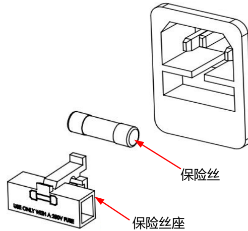
图 4.8 更换保险丝
