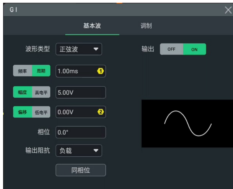
图 14.1 AFG 设置菜单
