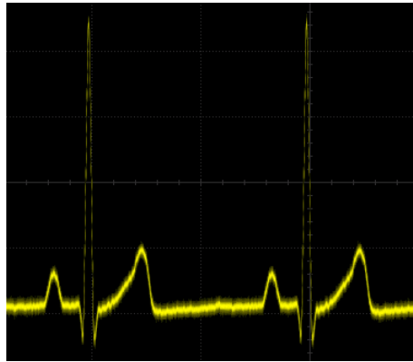
图 14.4 心电图
