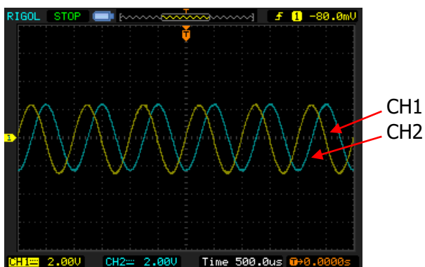
同相位前
