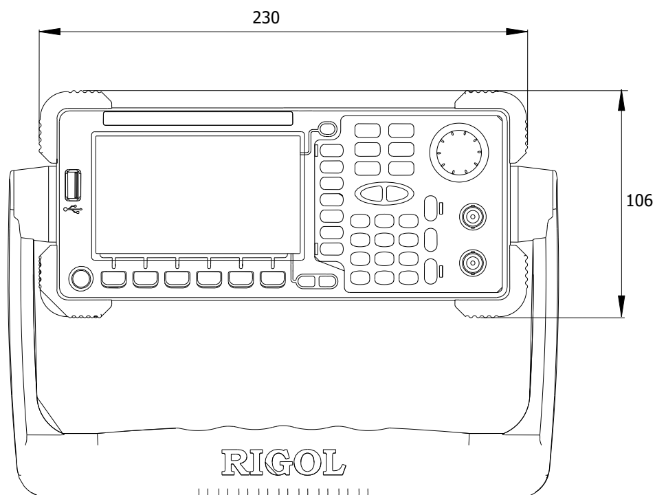
正视图
