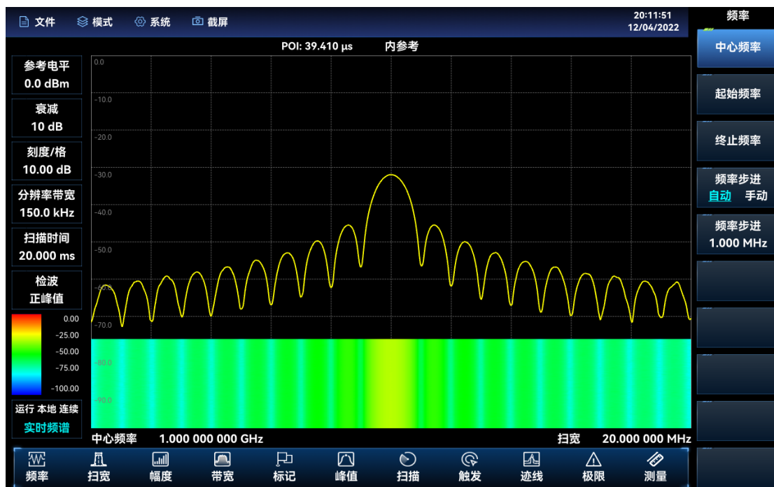
图 10.2 瀑布图示意图
