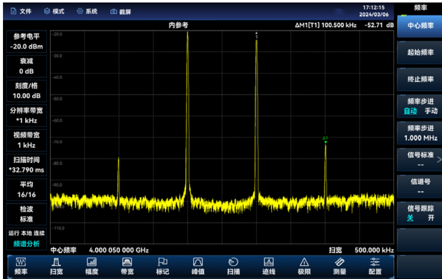
图 4.8 对内部调制失真进行相对测量
