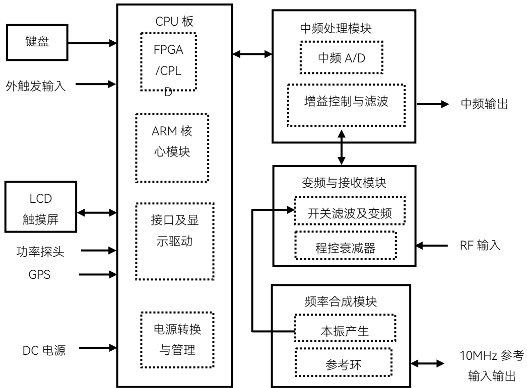
图 14.1 整机硬件总体方案框图
