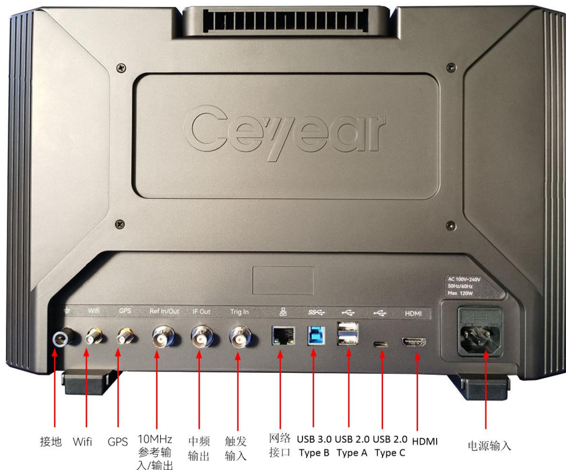
图 3.8 后面接口说明图
