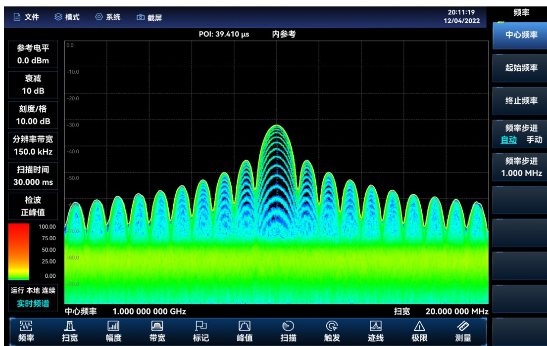
图 10.1 余辉图示意图
