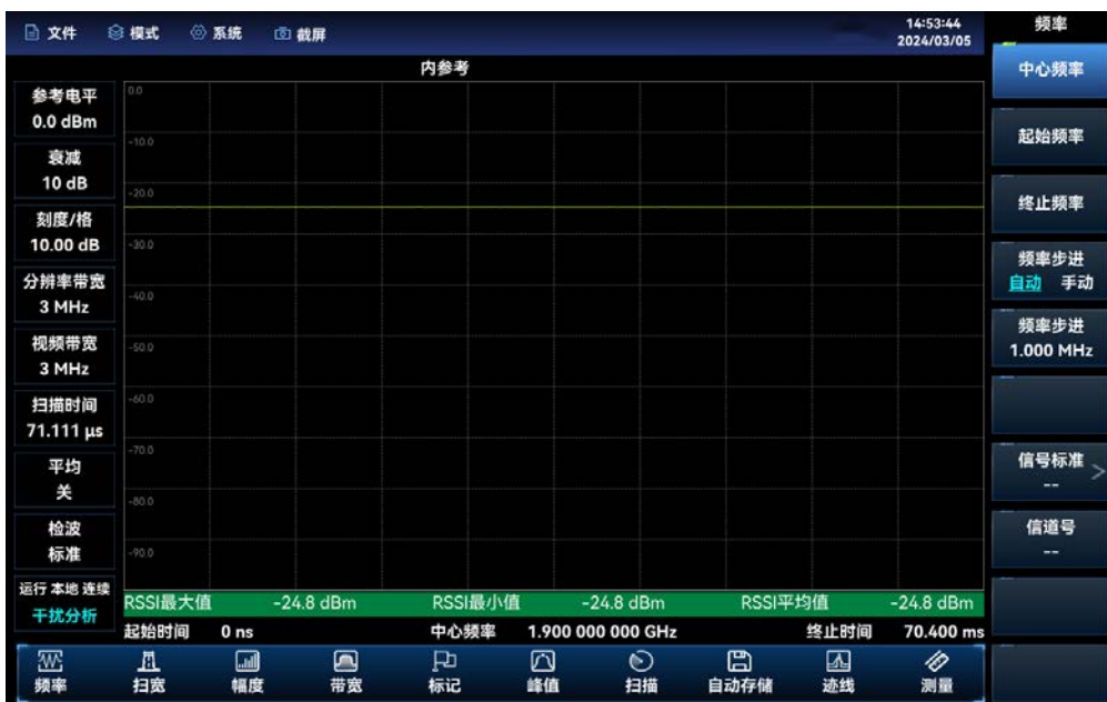
图 5.2 干扰分析 RSSI 测试图
