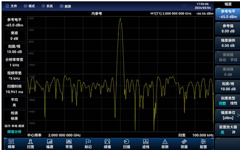
图 4.19 二次谐波幅度
