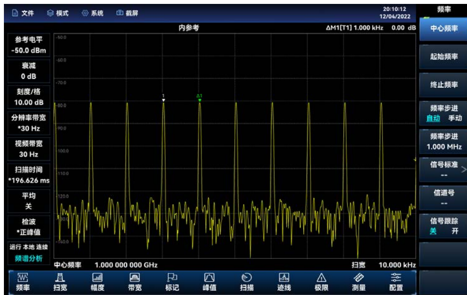
图 4.24 测量脉冲重复频率
