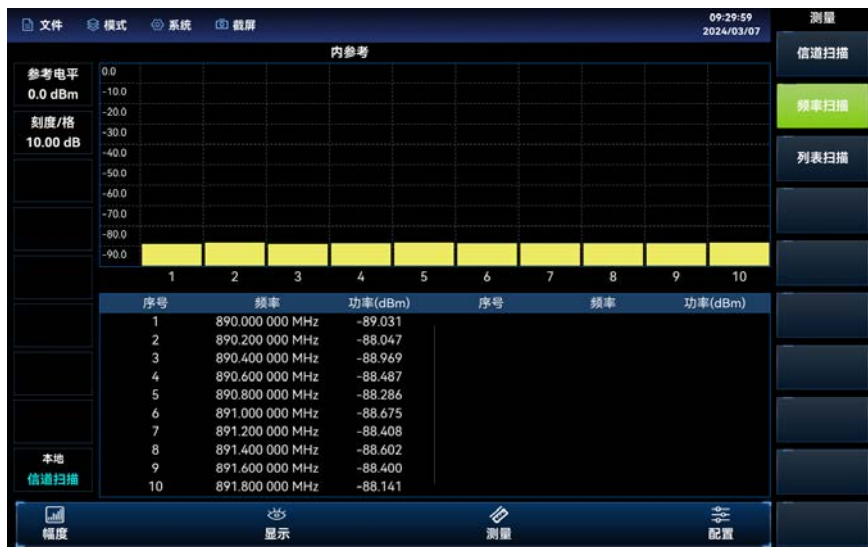
图 8.2 频率扫描模式界面图
