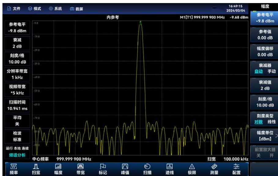
图 4.18 100kHz 扫宽下显示的输入信号
