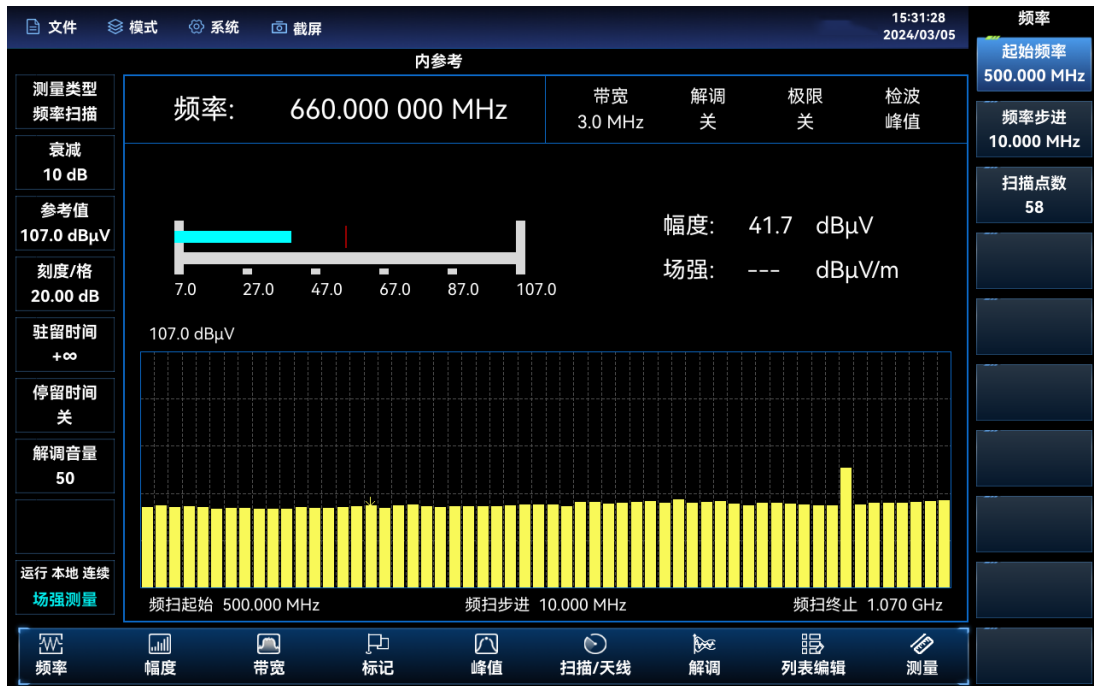
图 9.2 频率测量类型示意图
