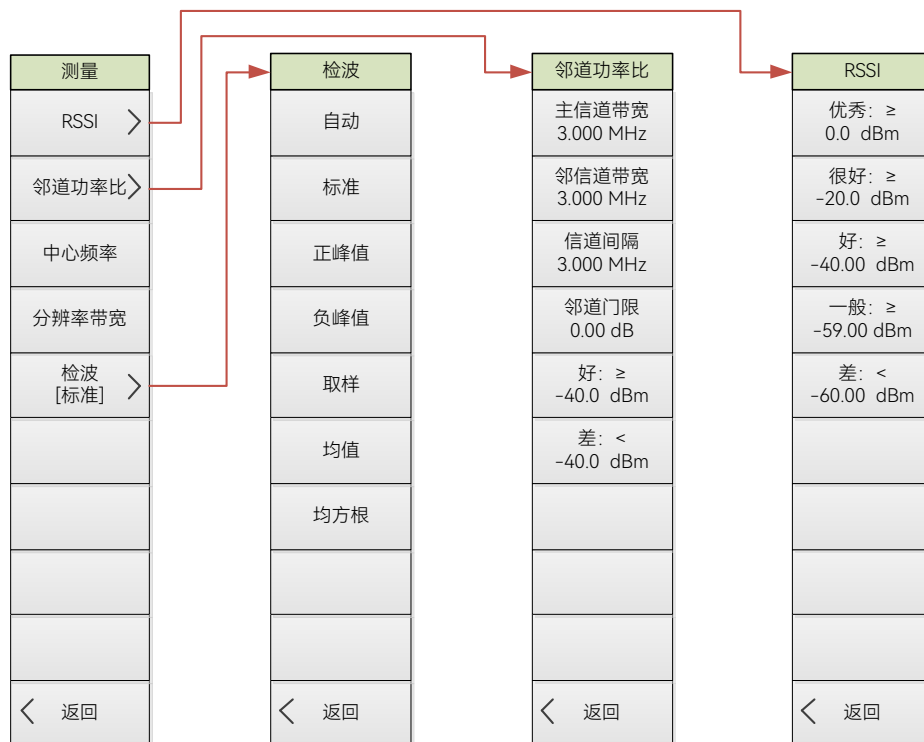
图 4.40 频谱分析模式测量菜单结构框图 (续 2)
