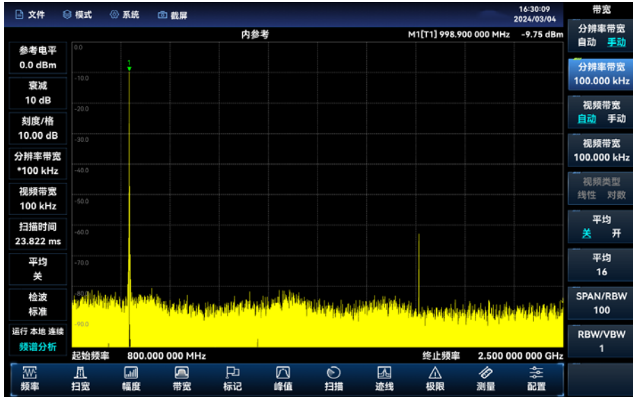
图 4.14 输入信号和谐波
