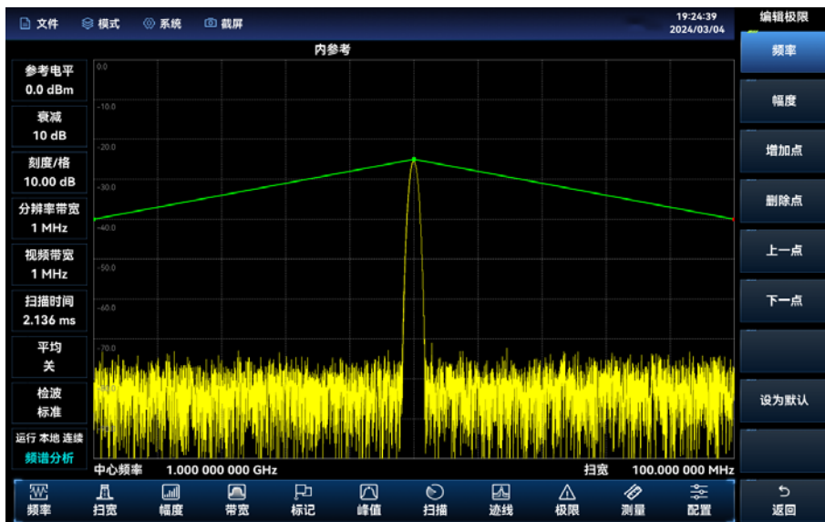
图 4.26 频谱发射模板测量
