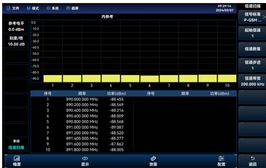
图 8.1 信道扫描模式界面图
