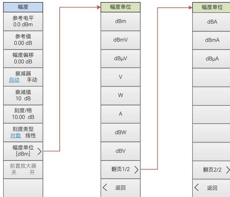
图 4.31 频谱分析模式幅度菜单结构框图
