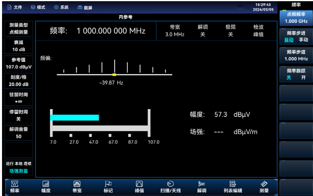
图 9.1 点频测量类型示意图
