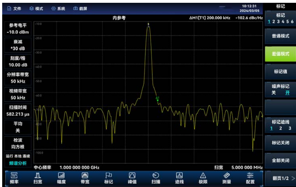
图 4.10 测量信噪比
