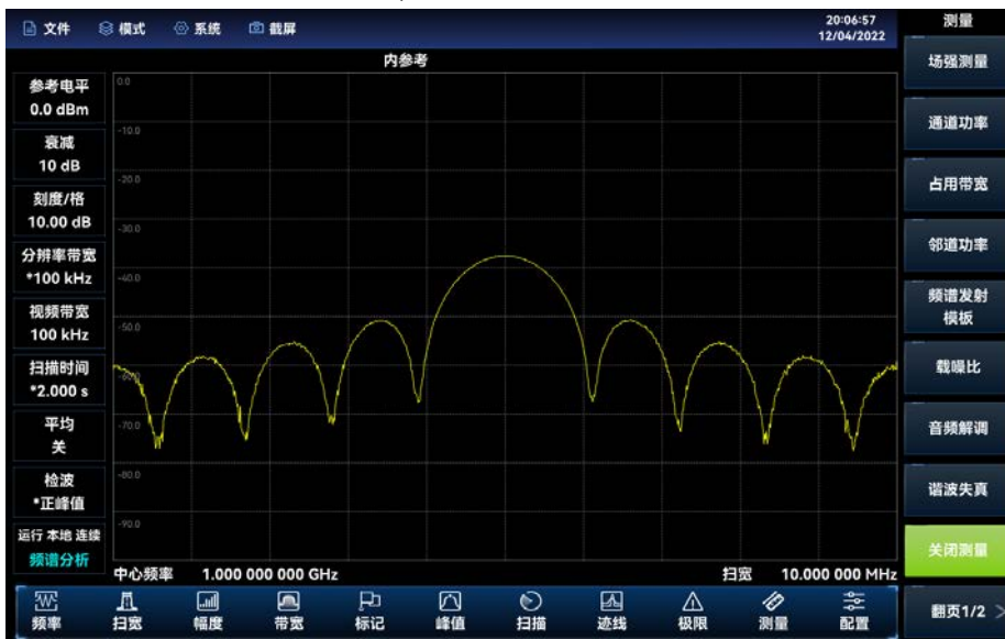
图 4.21 轨迹显示为实线
