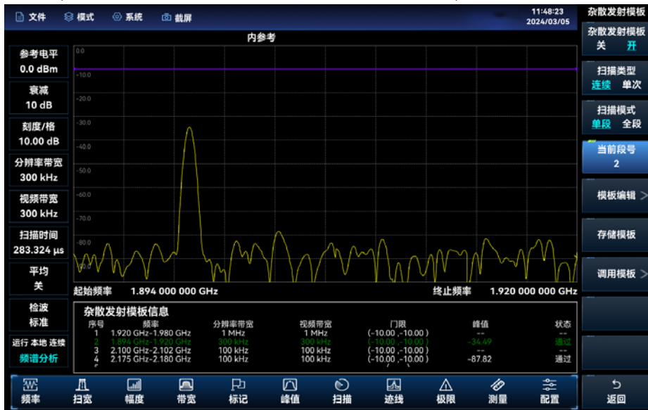
图 4.28 杂散发射模板测试
