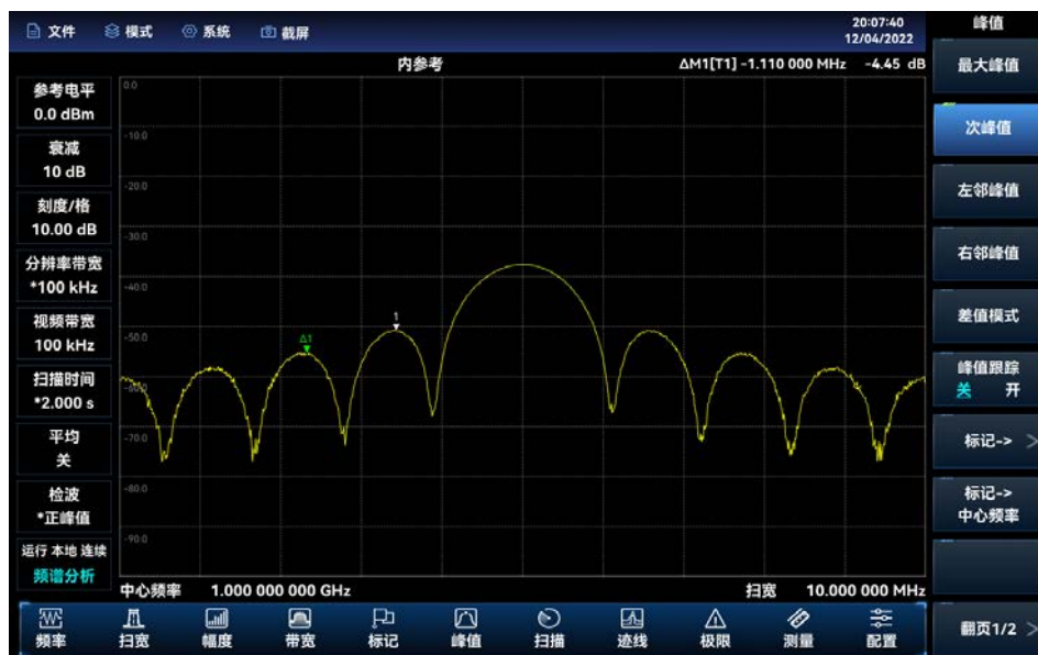
图 4.23 利用标记显示脉宽
