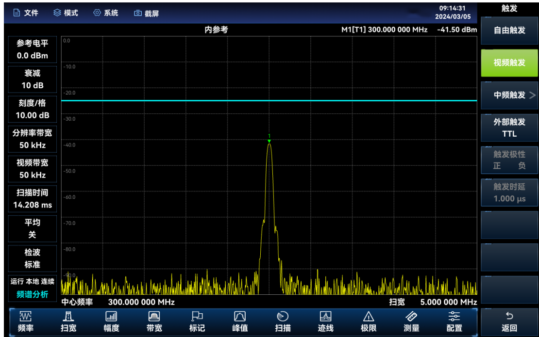
图 3.20 视频触发设置界面
