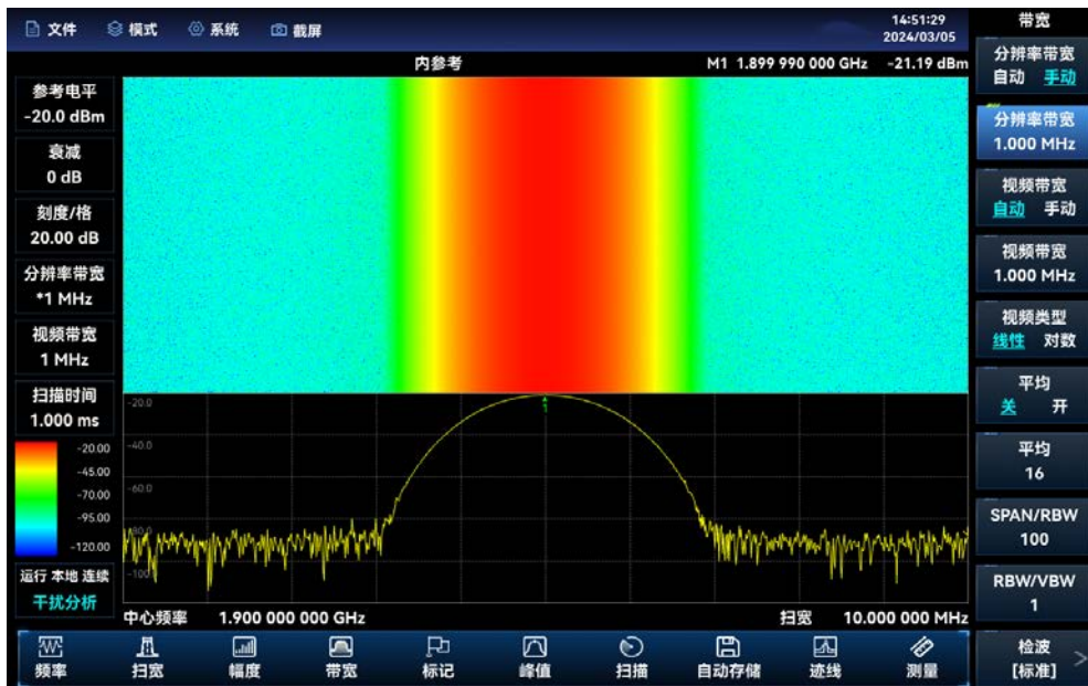
图 5.1 干扰分析瀑布图
