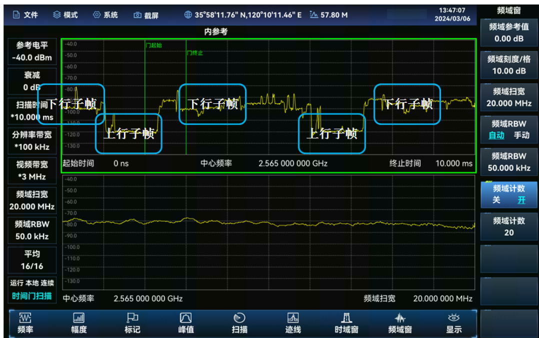
图 12.1 TDD 信号干扰排查示意图
