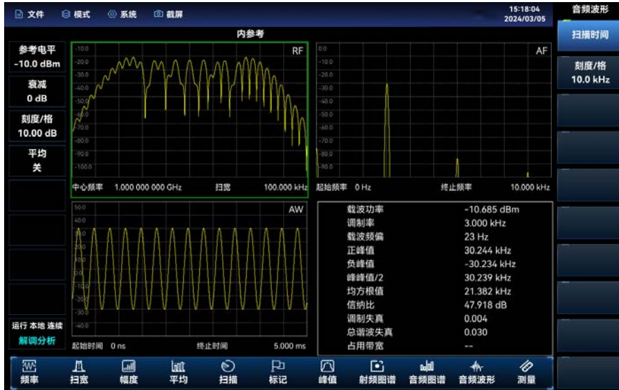
图 6.1 解调分析模式界面显示图
