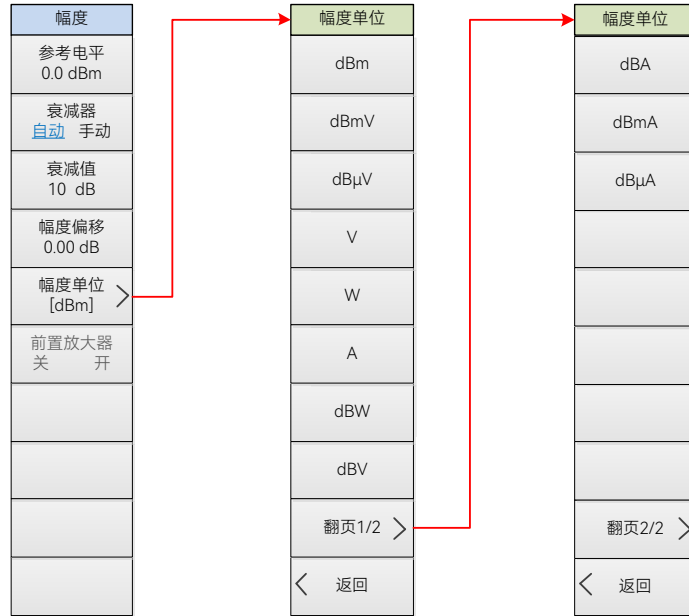
图 12.3 时间门扫描模式幅度菜单结构框图
