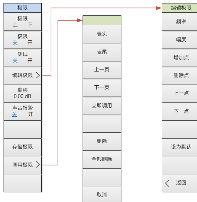
图 4.37 频谱分析模式极限菜单结构框图
