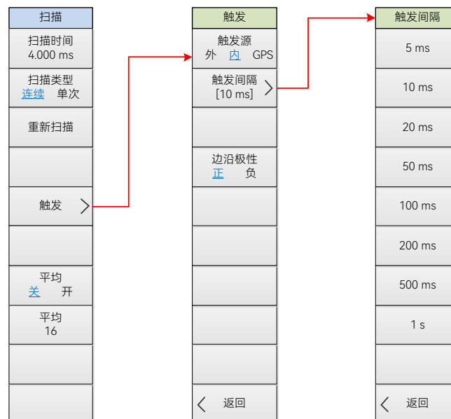
图 12.6 时间门扫描模式扫描菜单结构框
