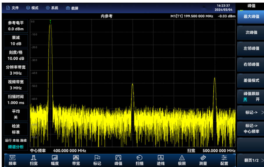
图 4.12 观测谐波失真
