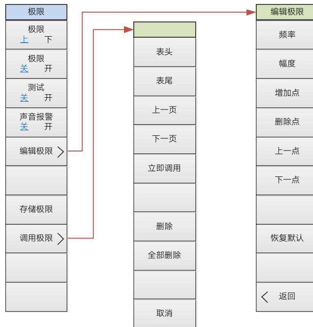
图 10.12 实时频谱模式极限菜单结构框图
