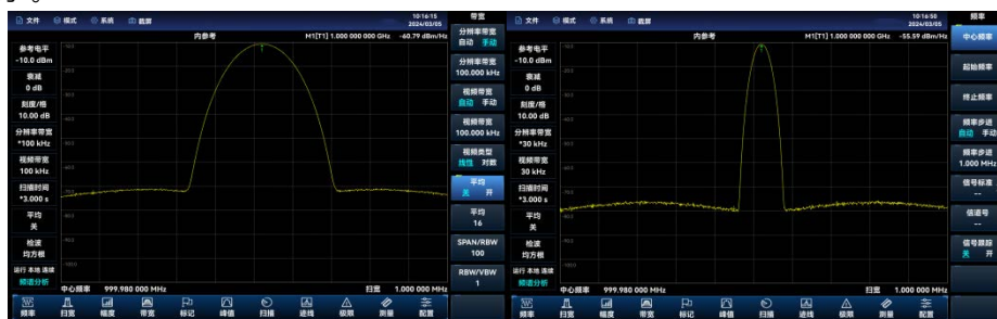
图 4.11 使用噪声标记功能测量噪声
