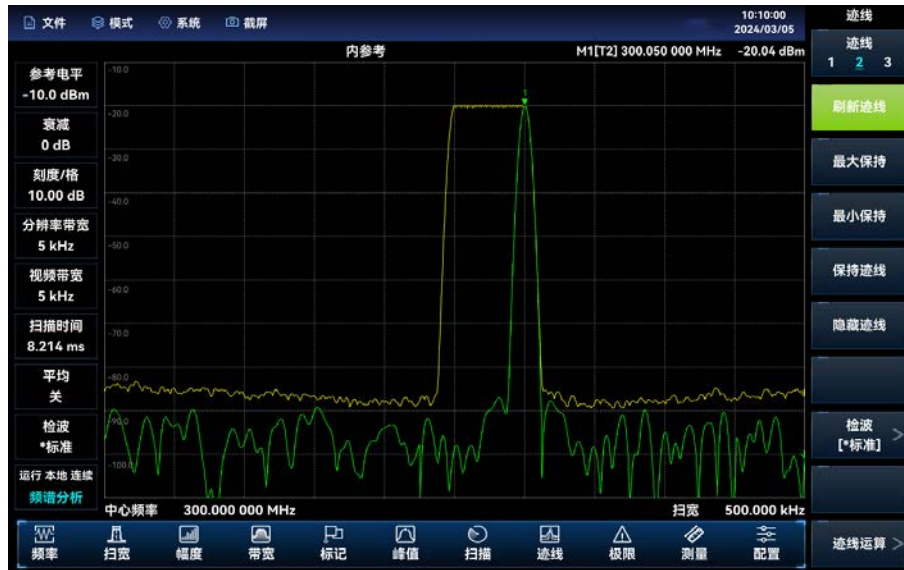
图 4.9 使用最大保持观测漂移信号
