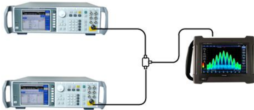
图 4.5 连接三阶交调失真测量系统
