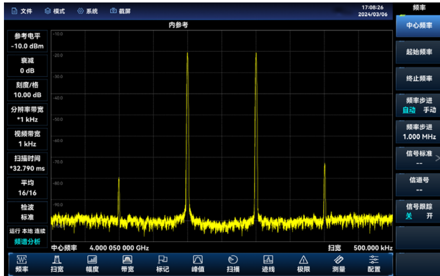
图 4.6 信号在频谱分析仪显示器中央
