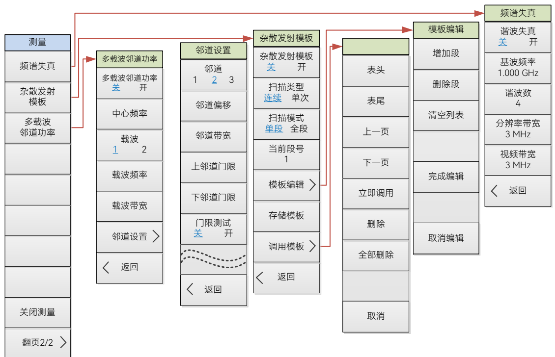
图 4.39 频谱分析模式测量菜单结构框图 (续 1)
