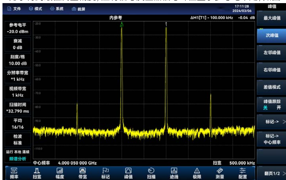
图 4.7 将信号峰值置于参考电平处
