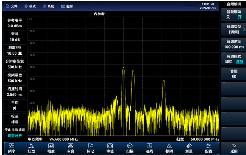
图 4.27 音频解调测试
