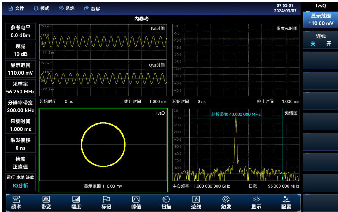
图 13.1 IQ 分析模式界面图
