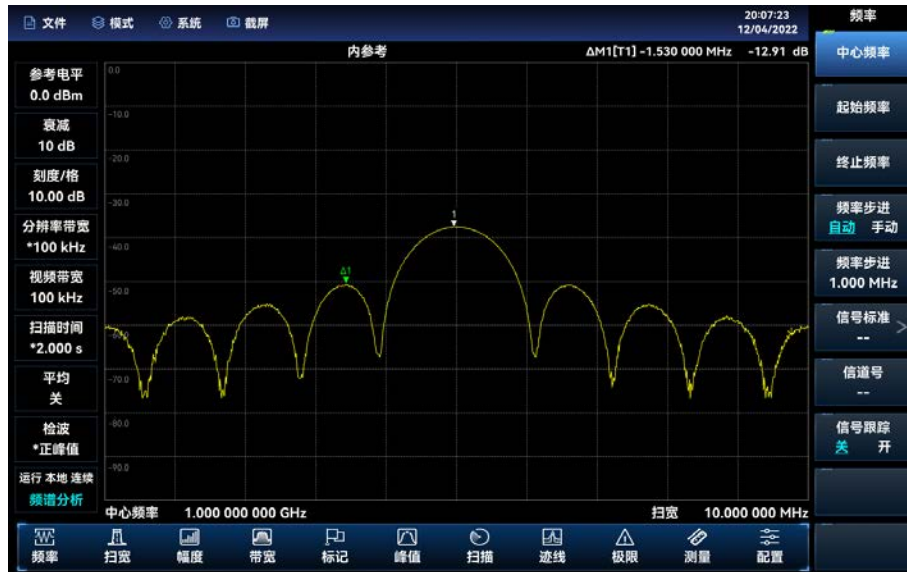
图 4.22 标记显示旁瓣比例
