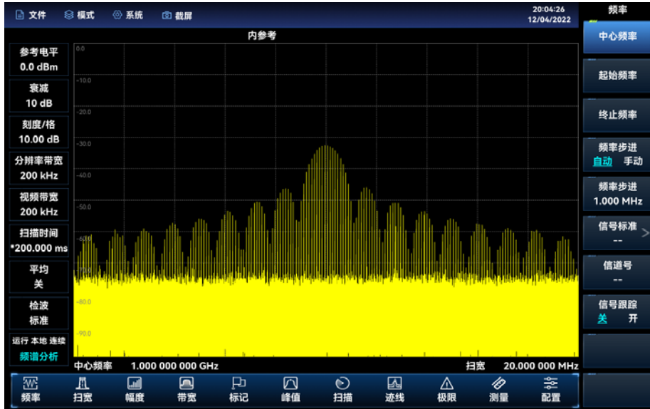
图 4.20 主瓣和旁瓣
