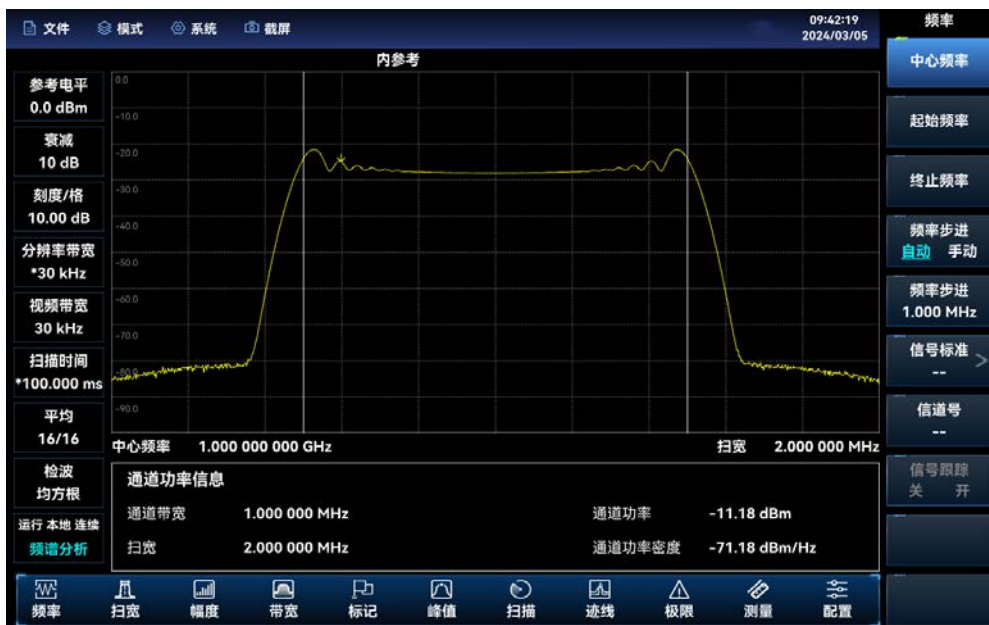
图 4.2 调频信号通道功率测量
