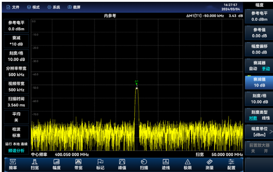
图 4.13 衰减器设置为 10dB
