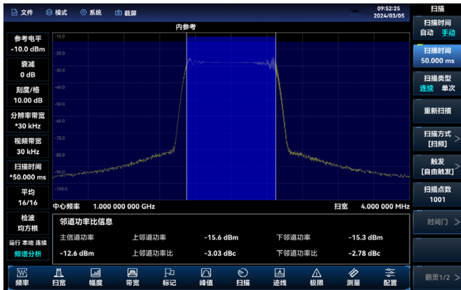
图 4.4 邻道功率比测量
